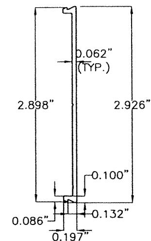
D SNAP PLATE (BATTEN) 6063-T6 Alum. ALLOY
